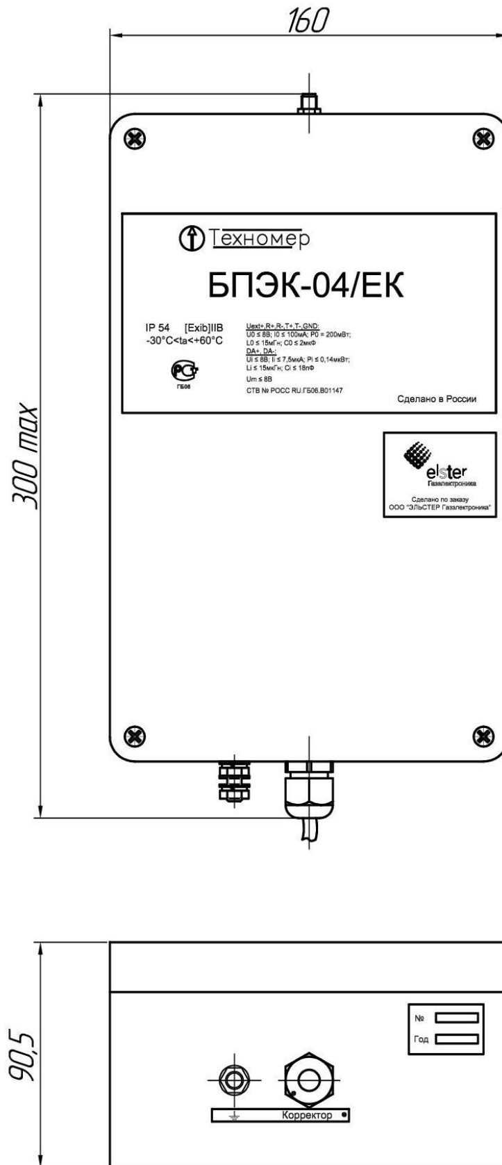
Рисунок 1 – Габаритные размеры модуля коммуникационного БПЭК-04/ЕК
